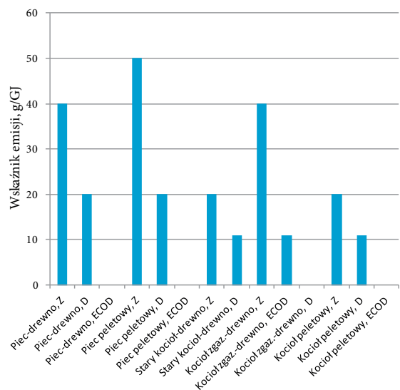
Rys. 18. Emisja zanieczyszczeń ze spalania drewna i pellet w różnych urządzeniach grzewczych Z – stara technika, D – nowa technika, ECOD – wymogi dyrektywy ErP
