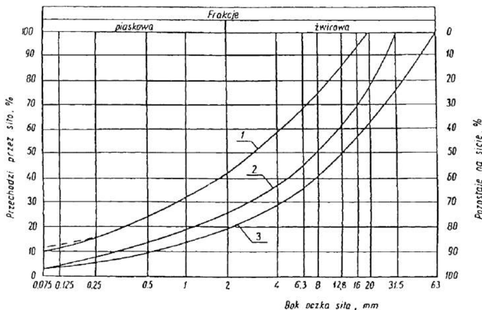
Rysunek 1. Pole dobrego uziarnienia kruszyw przeznaczonych na pobocze wykonywane metodą stabilizacji mechanicznej
