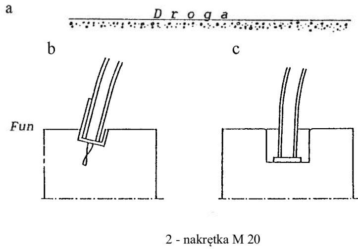
Załącznik 11 Przykład połączenia śrubami blach fali- stych 1 - śruba M 20
